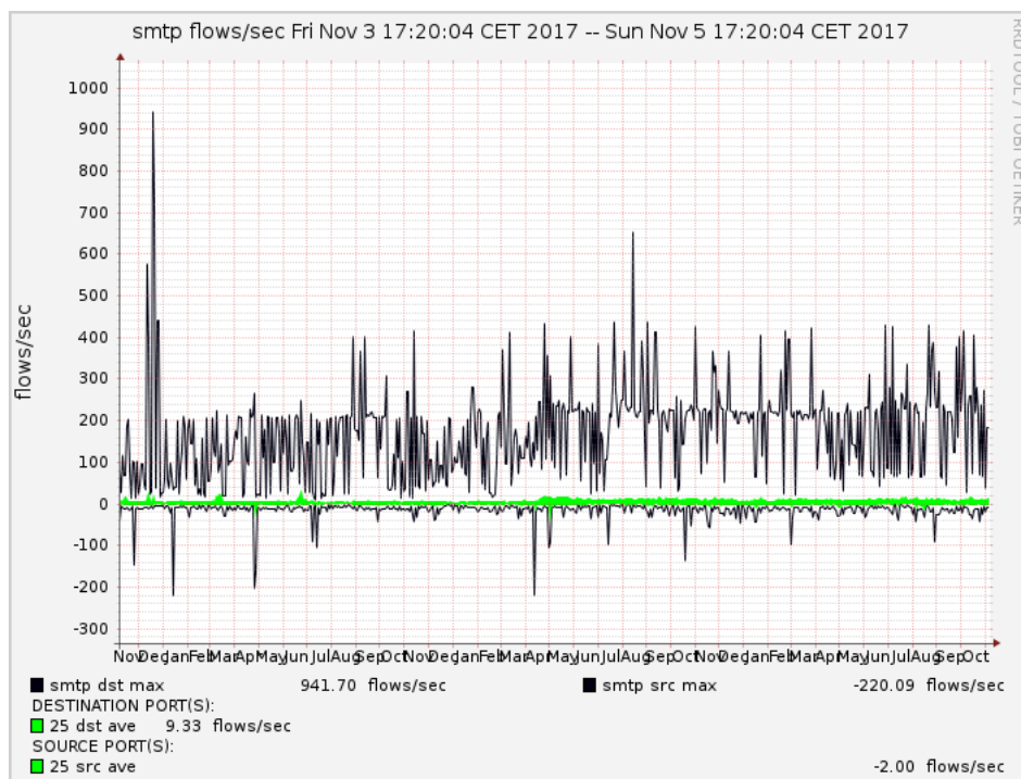
6. ábra. E-mail forgalom jellemző portja. Minden másodpercben érkezik közel 10 darab levél és minden másodpercben küldünk 2 levelet. A spam robotok kb. 200 levelet próbálnak küldeni másodpercenként.
